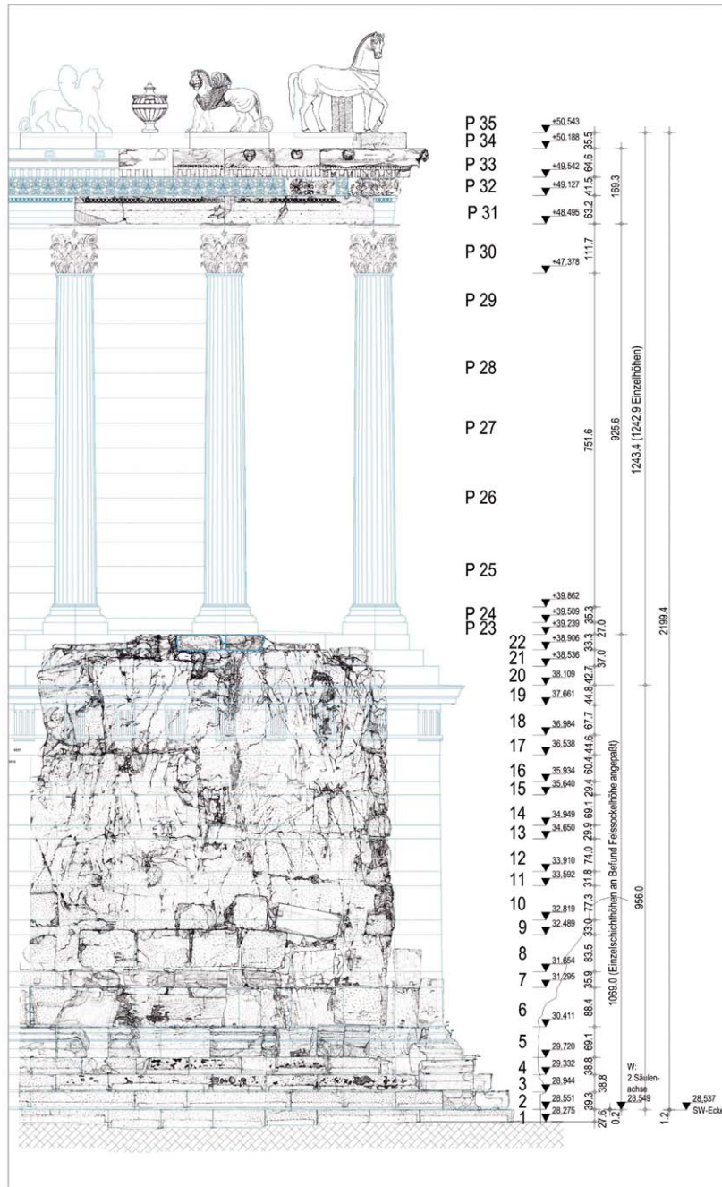
W-Fassade, Südteil Rekonstruktion mit Bestand M = 1 : 100.
