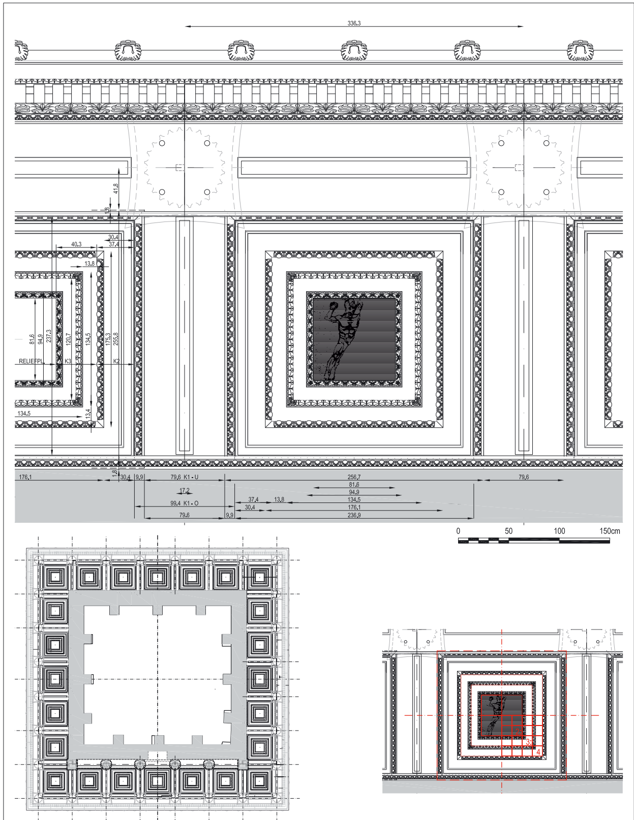
Deckenuntersicht Peristasis mit Kassetendecke M = 1 : 25, und Proportionsverhältnissen M = 1 : 50.
