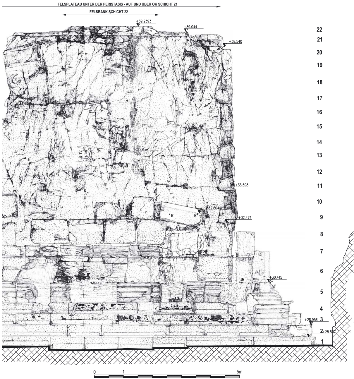
Südteil der Westfassade. Bestandsplan M = 1 : 50.
