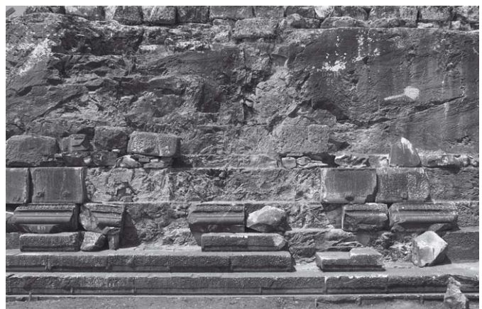
4: Klammernische der Südseite mit Schwalbenschwanz-Klammerloch; 5-7 Teilansichten der Ostwand mit Lagerflächeneinarbeitungen im Fels.
