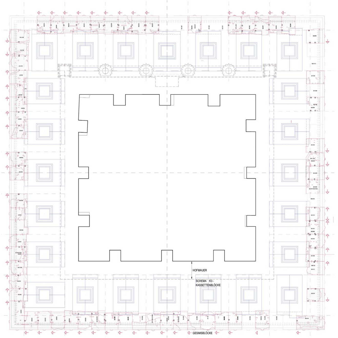
Gesimsblöcke der Peristasis und Lage der Kassettenblöcke K3 M = 1 : 100.
