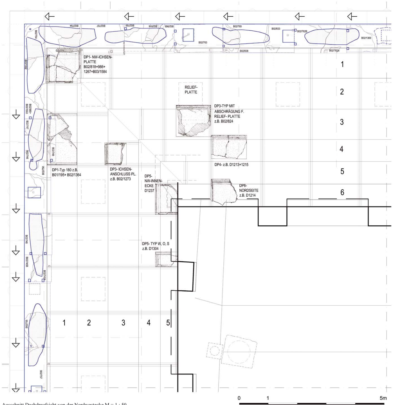
Ausschnitt Dachdraufsicht von der Nordwestecke M = 1 : 50.
